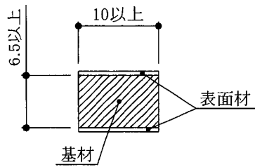
耐火マット用補助充填材断面図の一例
