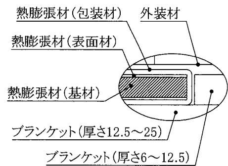
A部詳細
