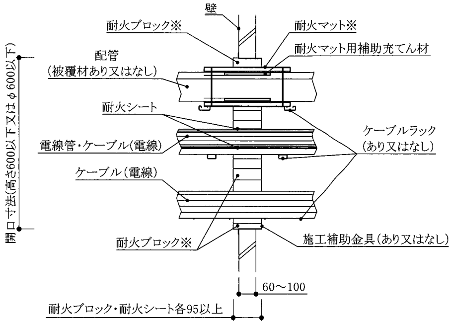
断面図 (壁厚が60以上, 100以下の中空壁以外の場合)
