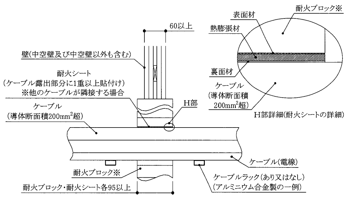
E-E断面図
