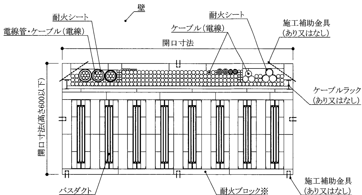
立面図(矩形の一例)
