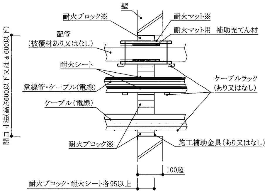
断面図 (壁厚が100を超える中空壁以外の場合)
