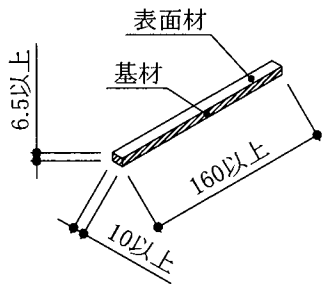
耐火マット用補助充填材詳細図の一例
